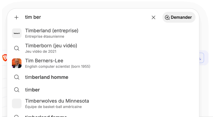
Fig. 3 : search.brave.com utilise Ajax pour faire de la complétion en temps réel.
